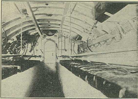
Akkumulatorrummet.
