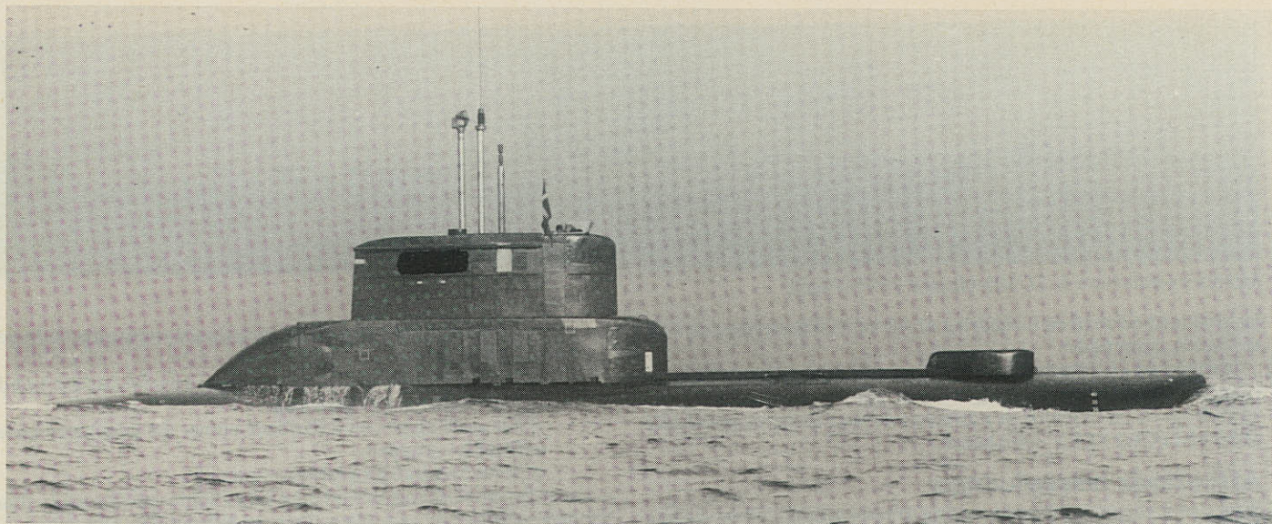
NARHVALEN-klassen. Længde: 44 m, bredde: 4,6 m, dybgang: 4,2 m, deplacement: 416 tons, fart: 14 knob. (SVN Foto).
