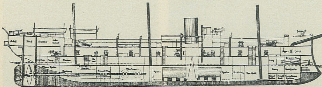
Delvis Plan (Batteri og Dæk).
